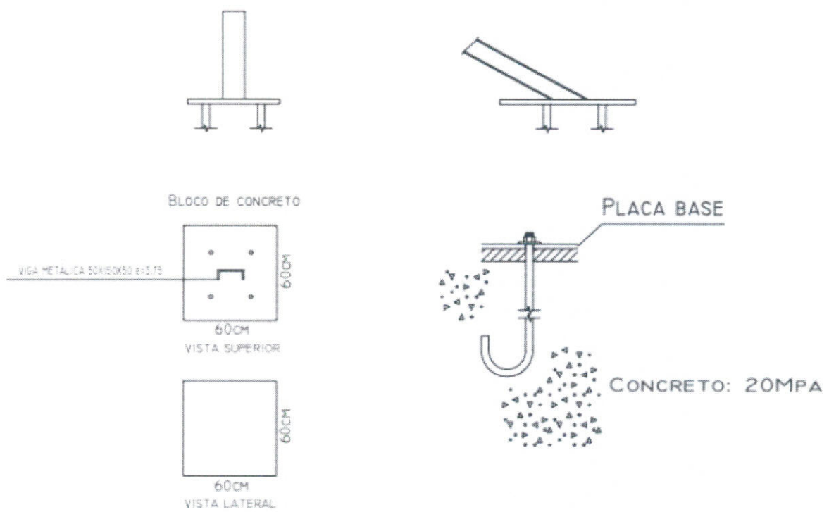
DETALHE ANCORAGEM VIGA INCLINADA E PILAR
