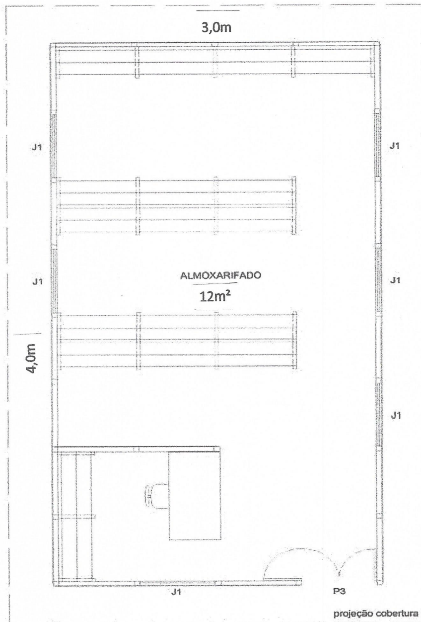
Figura 1 – Layout de referência de almojarifado em canteiro de obra, em chapa compensada, utilizado para fins de especificação.
