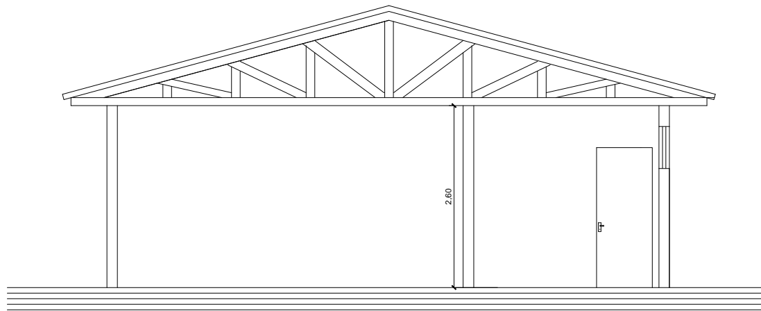
CORTE
